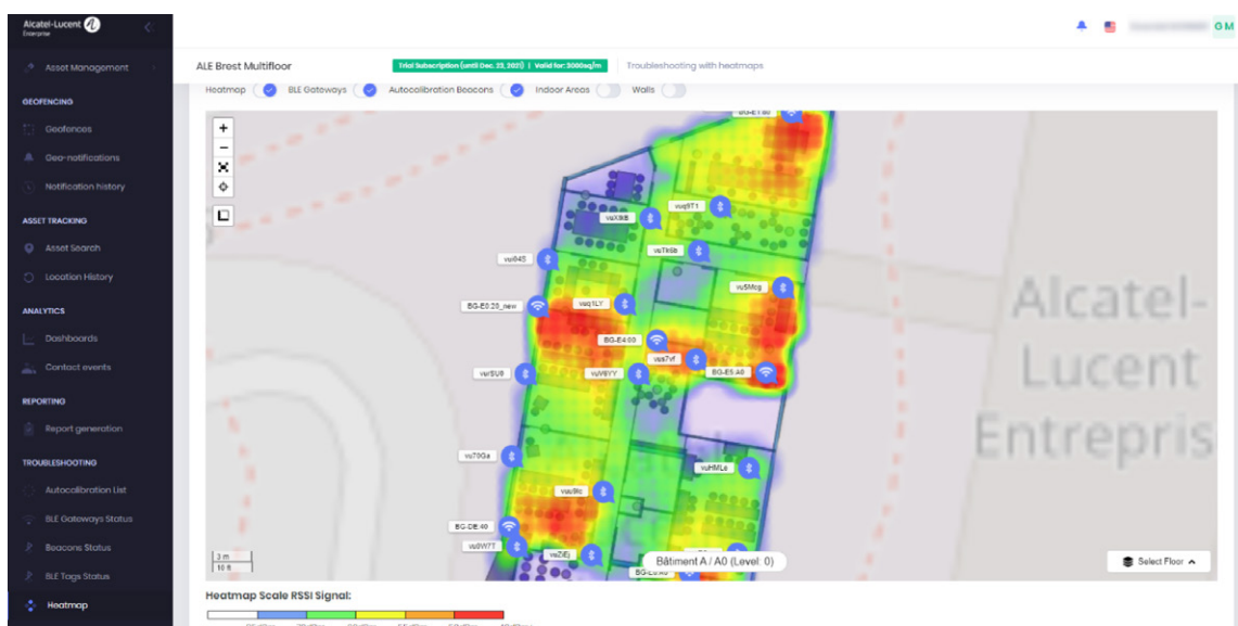
Figure 2. Validation du positionnement avec ALE Asset Tracking Manager (Plateforme de gestion dans le Cloud)
