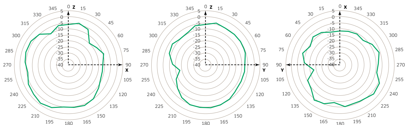
Abbildung 1. OmniAccess AP1201 BLE-Antennenmuster
