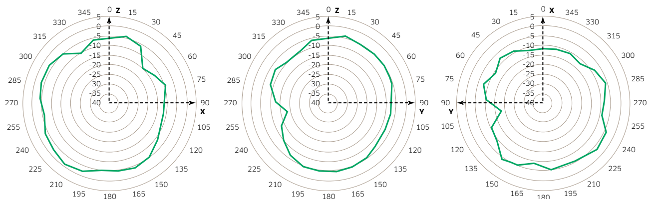
Figure 1. Tracés de modèles d'antenne BLE OmniAccess AP1201
