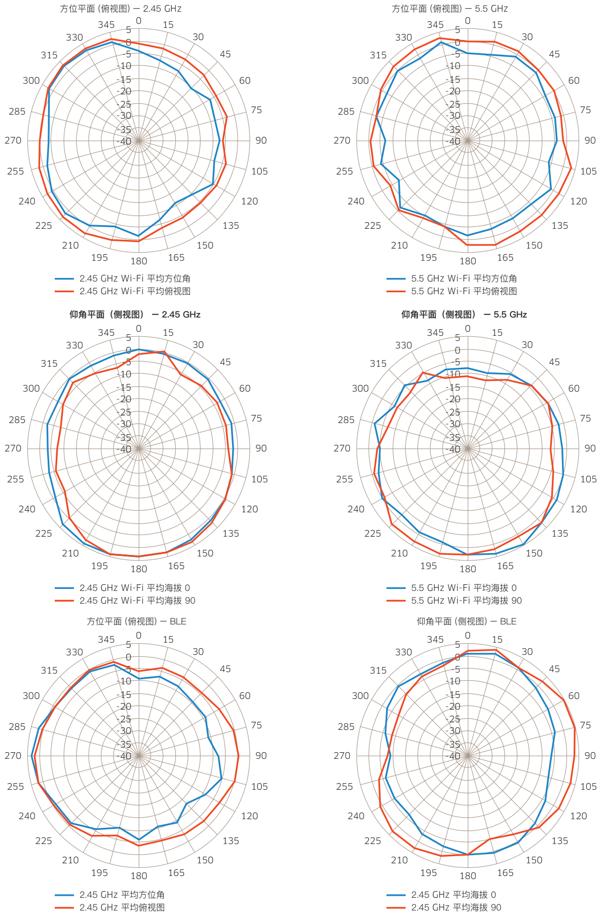
图. OmniAccess AP1311 天线模式图
