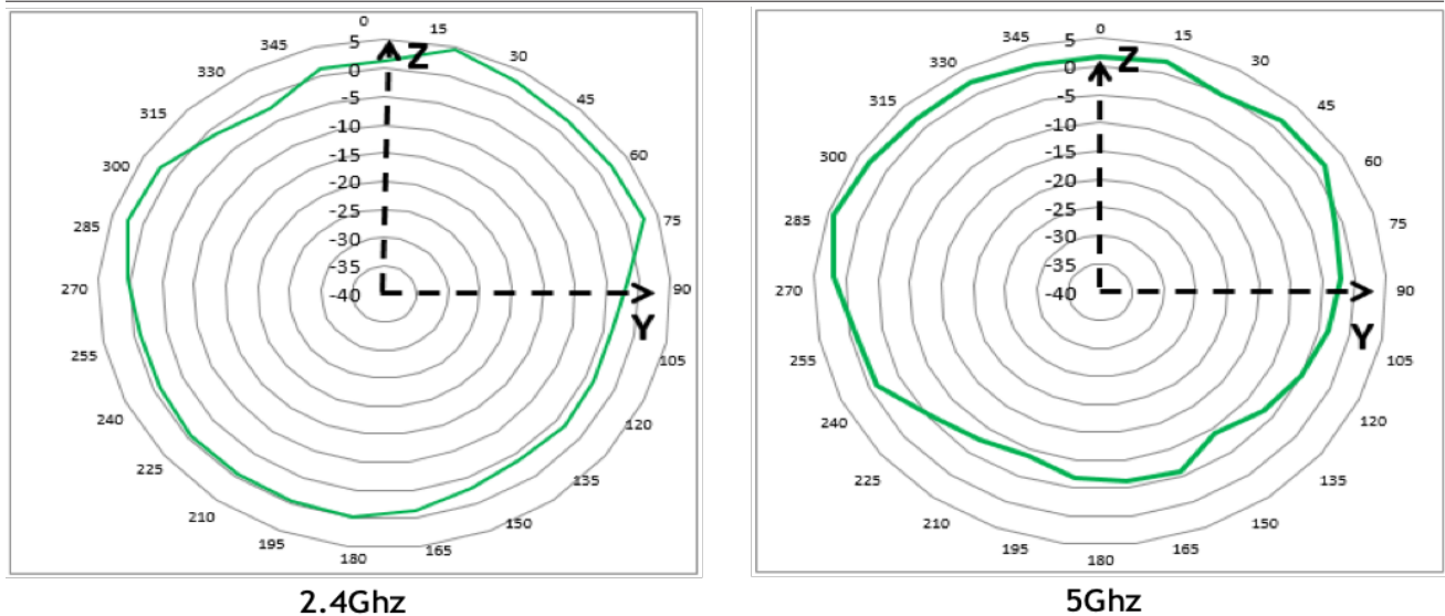
仰角平面（侧视图，0度角）
