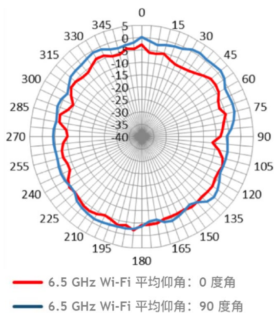
方位平面(顶视图) - 6GHz
