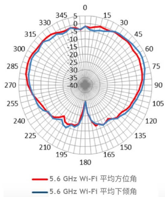
仰角平面(侧视图) - 5GHz
