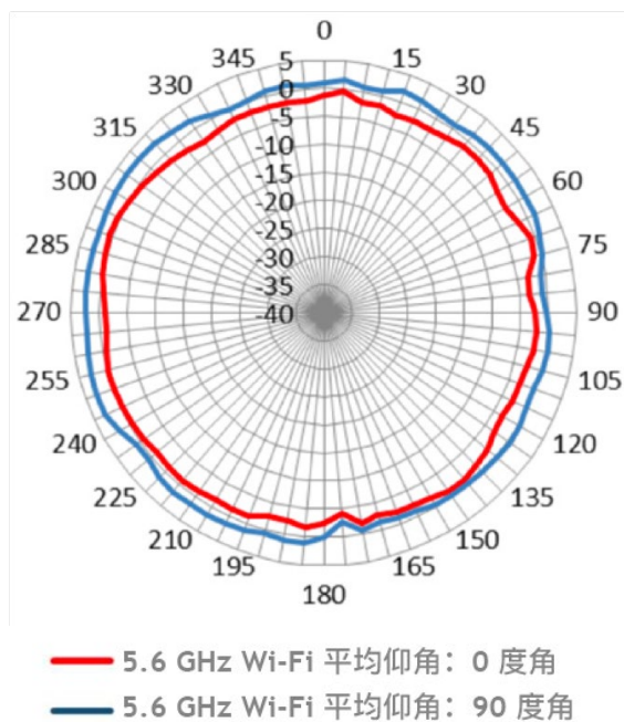
方位平面(顶视图) - 5GHz
