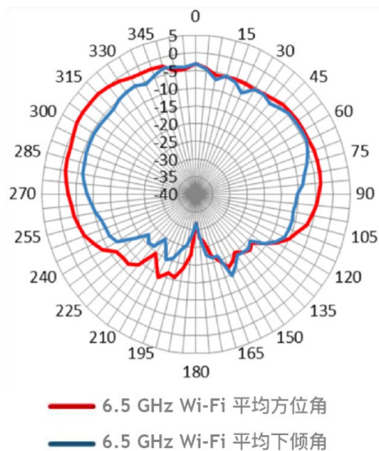
仰角平面(侧视图) - 6GHz
