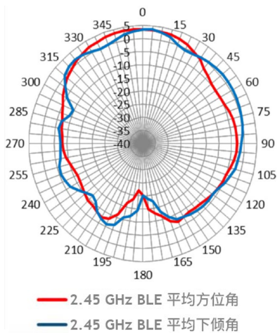
仰角平面(侧视图) - BLE
