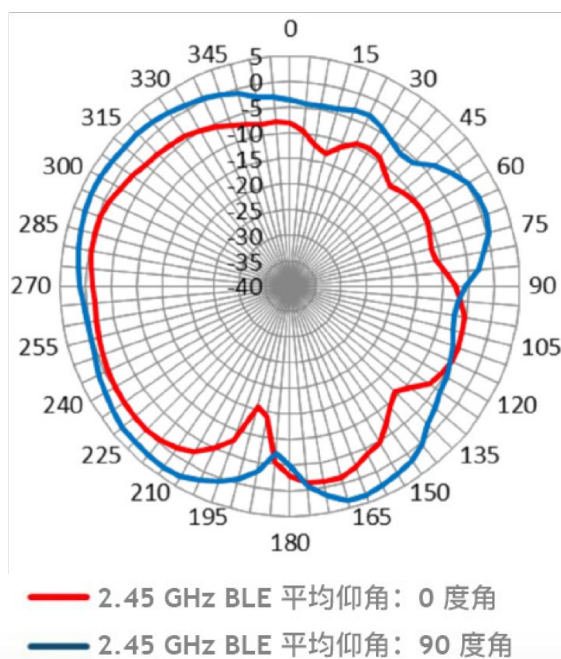
方位平面(顶视图) - BLE
