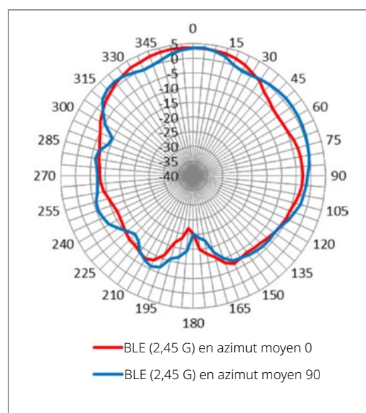
Plan d'élévation (vue de côté) - BLE
