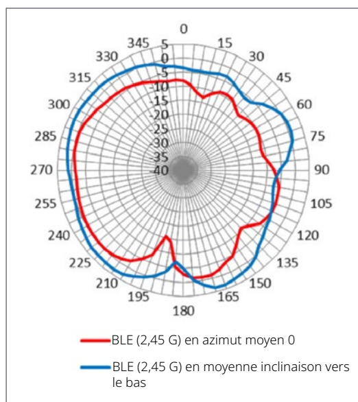
Plan azimut (vue du haut) - BLE
