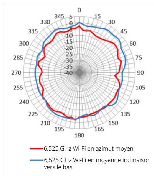
Plan azimut (vue du haut) - 6 GHz
