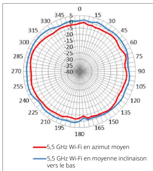
Plan azimut (vue du haut) - 5 GHz
