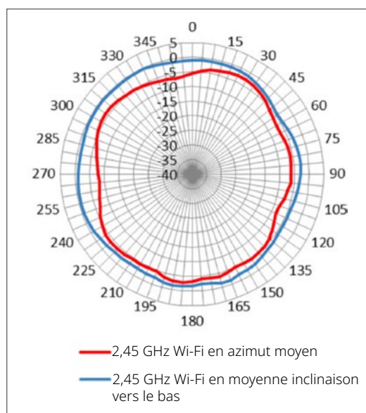
Plan azimut (vue du haut) - 2,4 GHz
