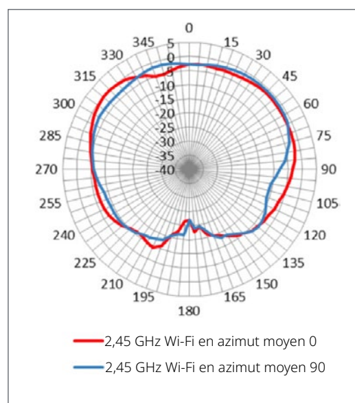
Plan d'élévation (vue de côté) - 2,4 GHz
